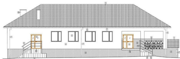
Elewacja północna (frontowa)
