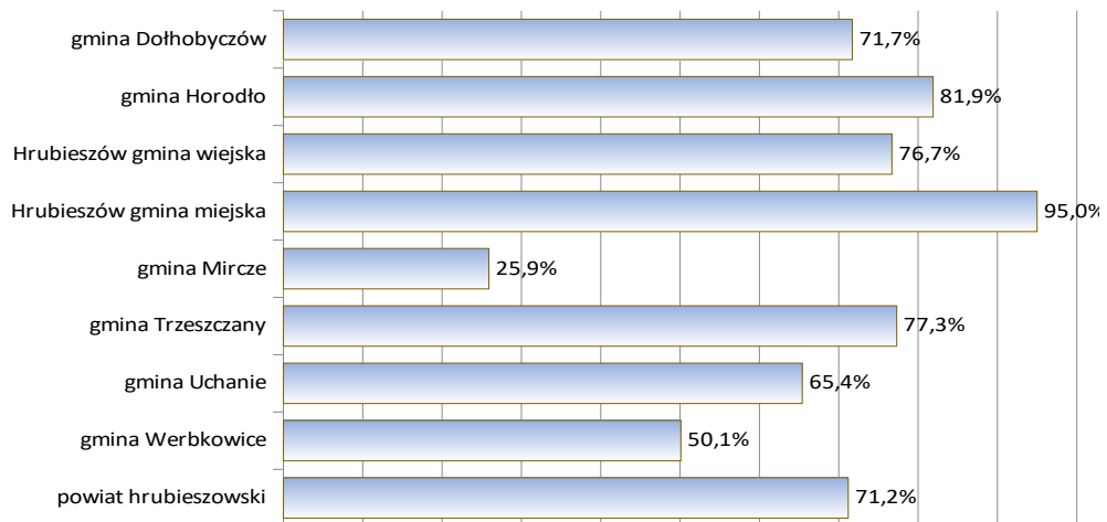
Wykres 22 Korzystający z sieci wodociągowej w % ogółu ludności w gminach powiatu hrubieszowskiego w 2022 roku
