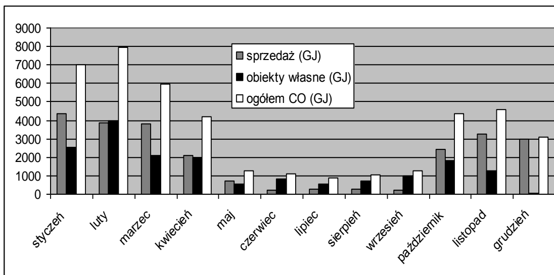
Rysunek 4.7. Produkcja energii cieplnej na cele grzewcze w budynkach w elektrociepłowni przemysłowej Cukrowni Werbkowice
